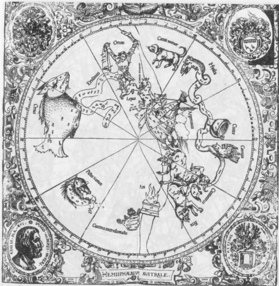
Рис. 3.3. Звездна карта на южното полукълбо, направена от А. Дюрер (1471–1528), уж през 1527 г. От [90], с. 9.
