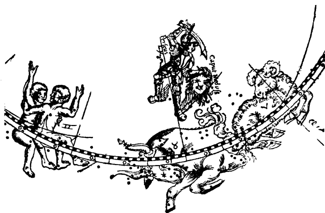
Рис. 3.33. Съзвездията Персей, Близнаци и Телец в звездната карта на Птолемеевия Алмагест. Увеличен фрагмент от картата. Отстранихме другите съзвездия, за да не претрупваме рисунката. От книгата на Claudii Ptolemaei „Pelusiensis Alexandrini omnia quae extant opera“, 1551 г., [1073]. Книгохранилището на Пулковската обсерватория (Санкт Петербург). Вж. също [543], между с. 216–217.
